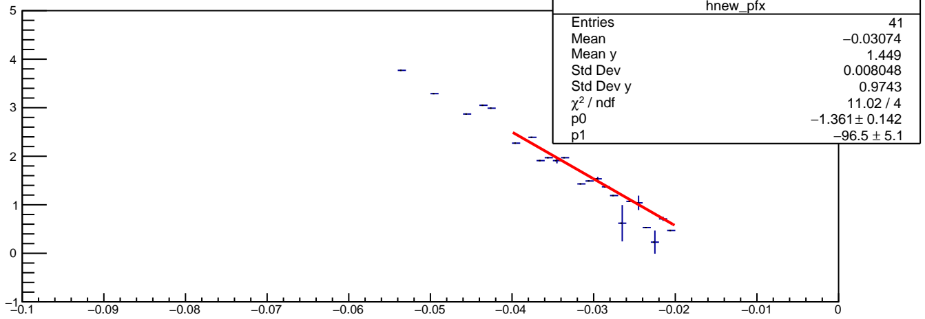
fspTrkZ0:fspPY/fspP {!fspHasL1&&fspMatchChisq<5&&fspTrkChisq<25}
