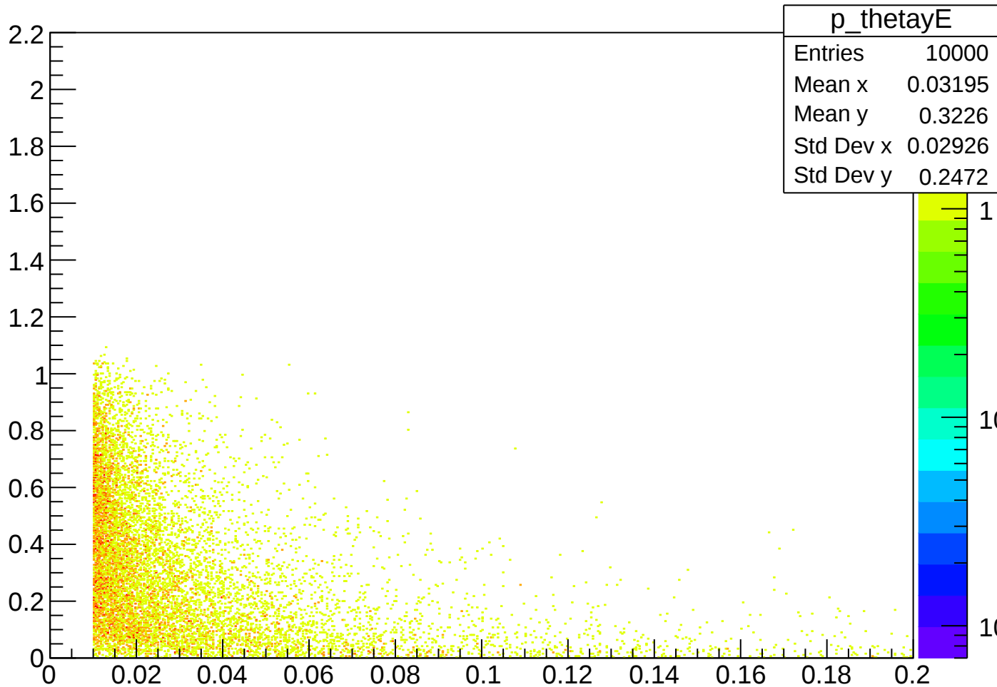
positron E vs. theta_y
