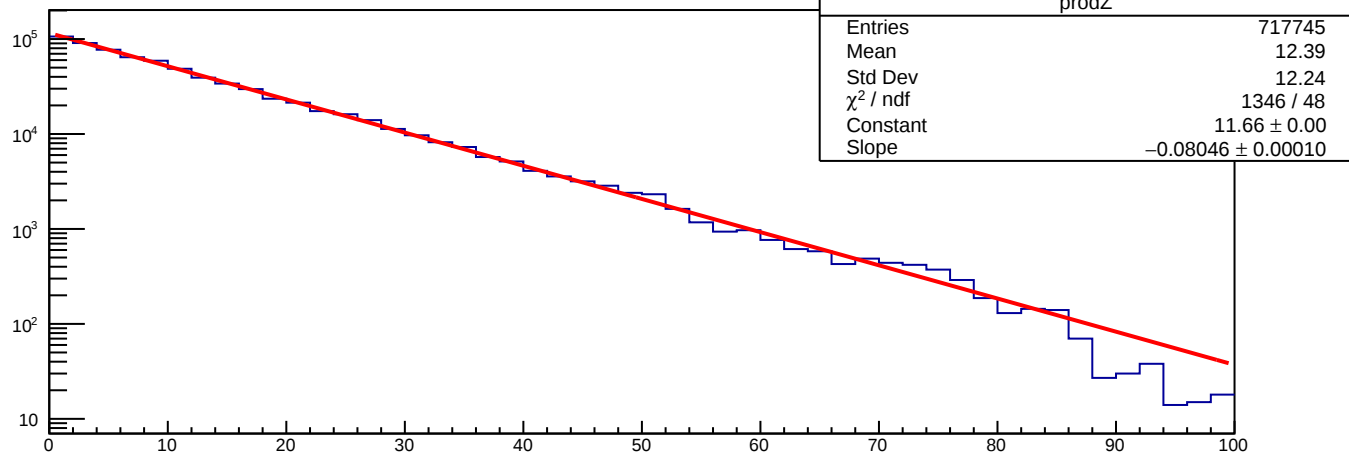
triEndZ {triP&gt;0.8*1.056}
