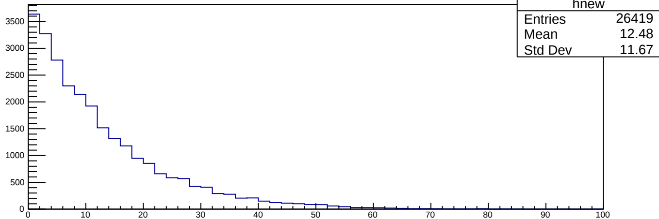
triEndZ {triP>0.8*1.056&&bscP>0.8*1.056}
