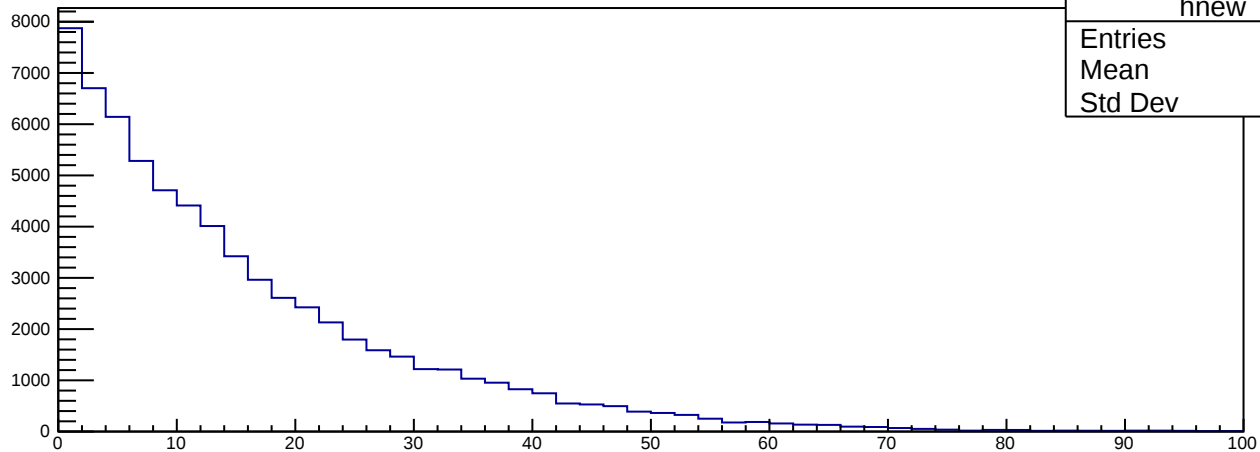
triEndZ {triP>0.8*1.056&&bscP>0.8*1.056}
