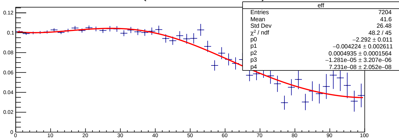
triEndZ {triP>0.8*1.056&&bscP>0.8*1.056}
