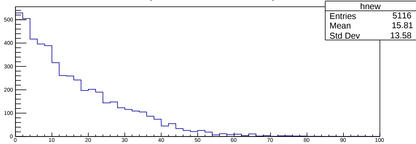
triEndZ {triP>0.8*1.056&&bscP>0.8*1.056}
