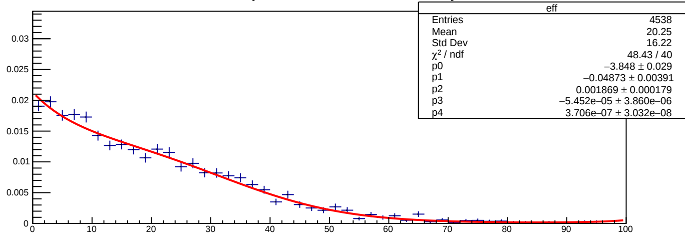
triEndZ {triP>0.8*1.056&&bscP>0.8*1.056}
