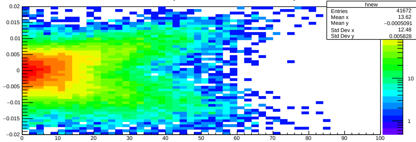
uncM-triM:triEndZ {triP>0.8*1.056&&bscP>0.8*1.056}
