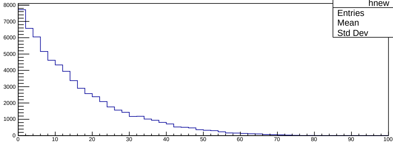
triEndZ {triP>0.8*1.056&&bscP>0.8*1.056}
