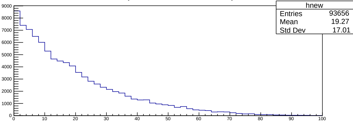
triEndZ {triP>0.8*1.056&&bscP>0.8*1.056}
