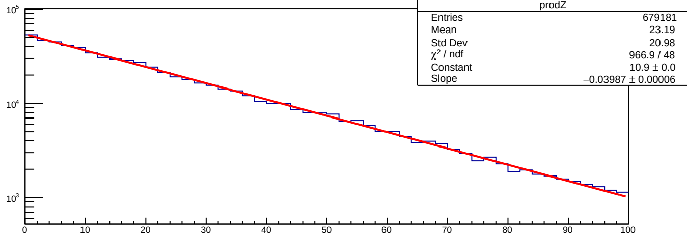
triEndZ {triP&gt;0.8*1.056}
