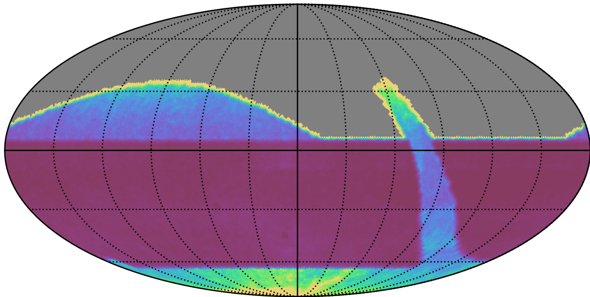
tmsd10 : properMotion
