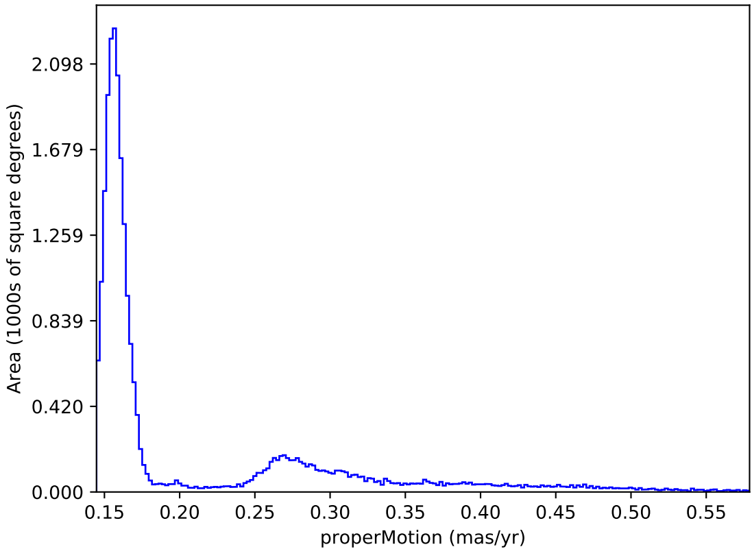
tmsd10 : properMotion
