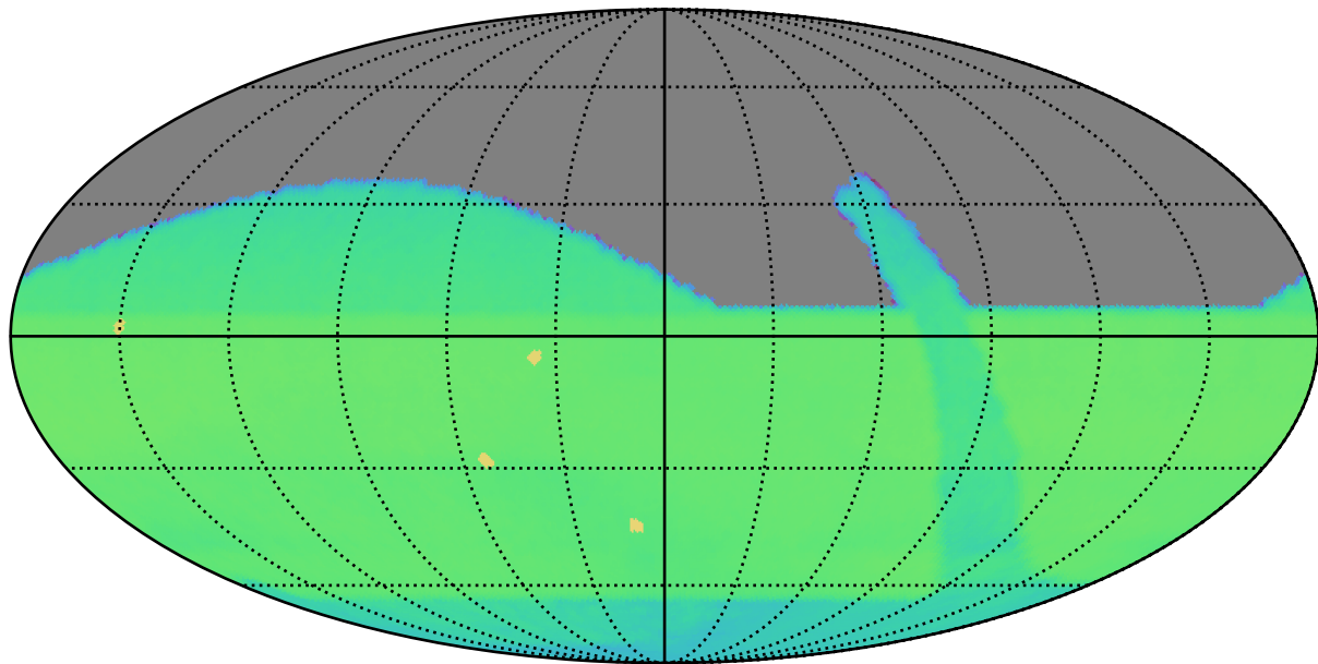
tmsd10 : CoaddM5
