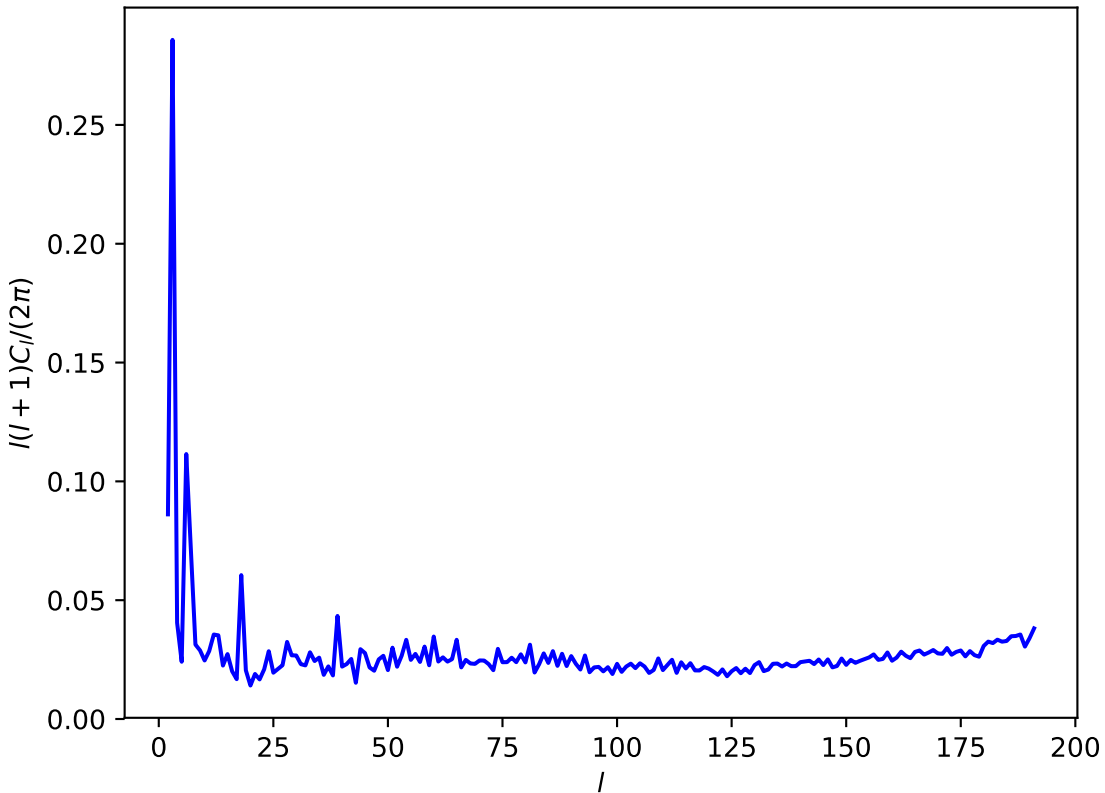
tmsd10 : CoaddM5
