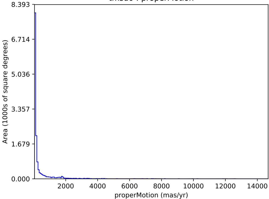
tmsd0 : properMotion
