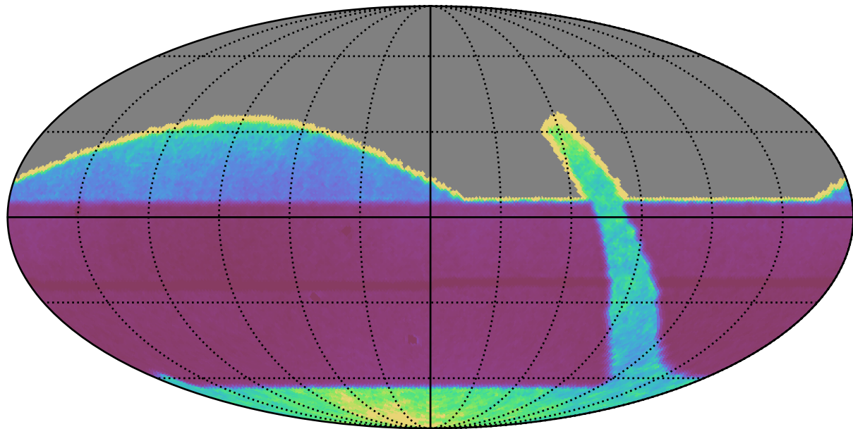
rolling10 : properMotion
