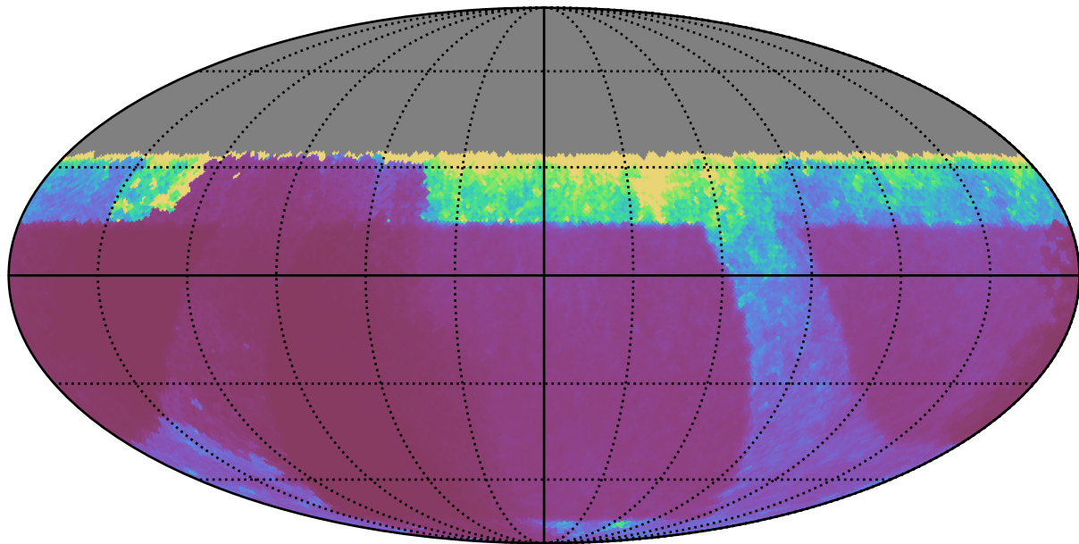
newwfdnodd : properMotion
