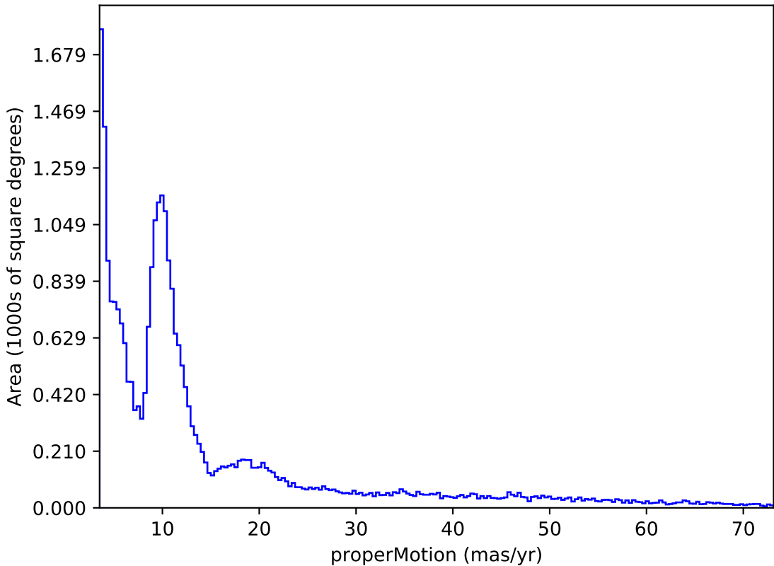
newwfdnodd : properMotion
