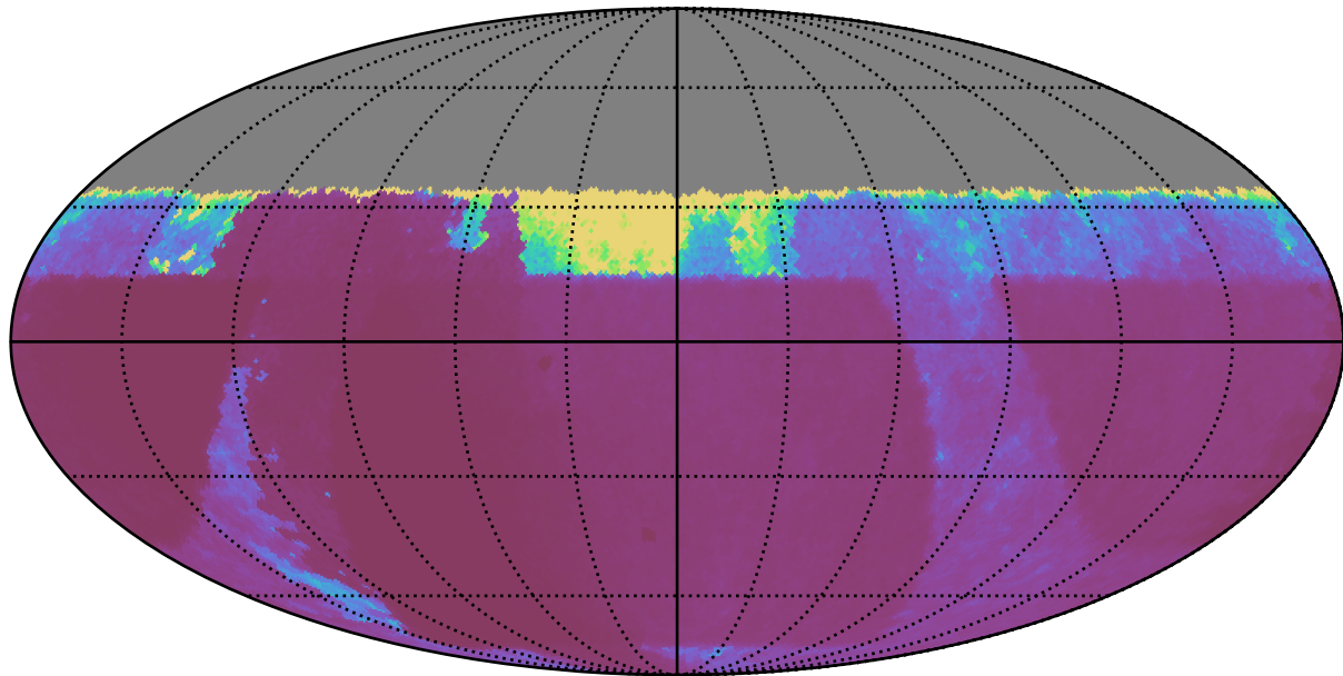
newwfd0 : properMotion
