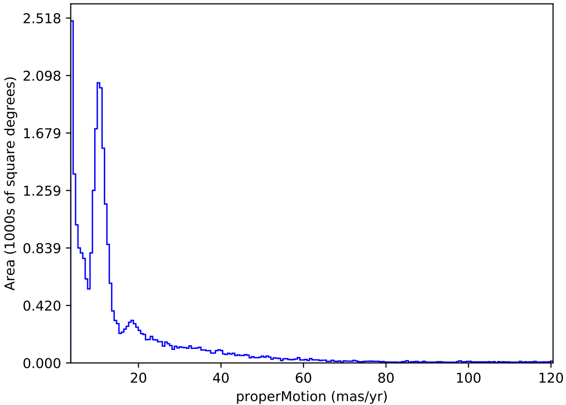
newwfd0 : properMotion
