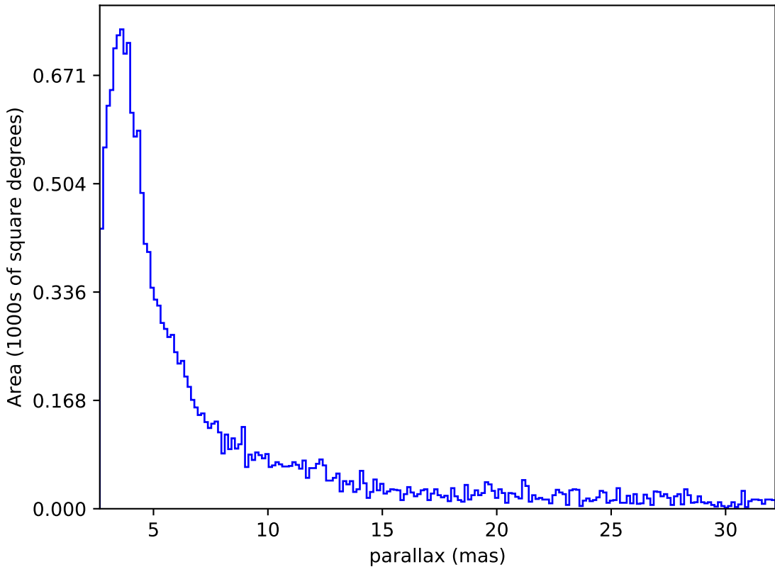
newwfd0 : parallax
