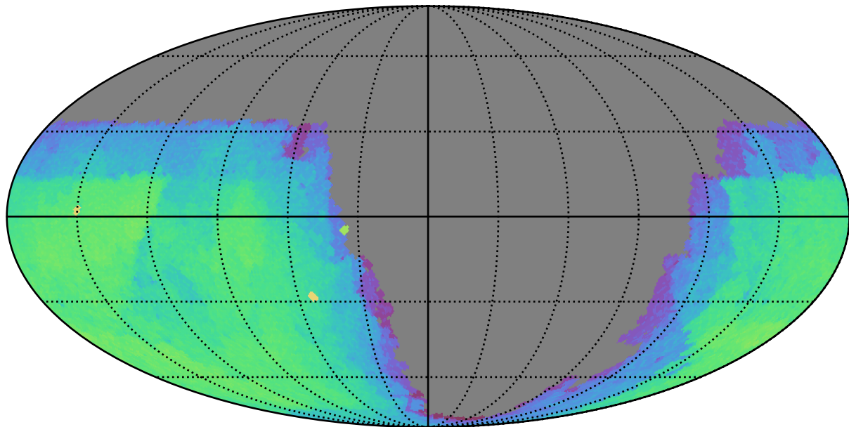
newwfd0 : CoaddM5
